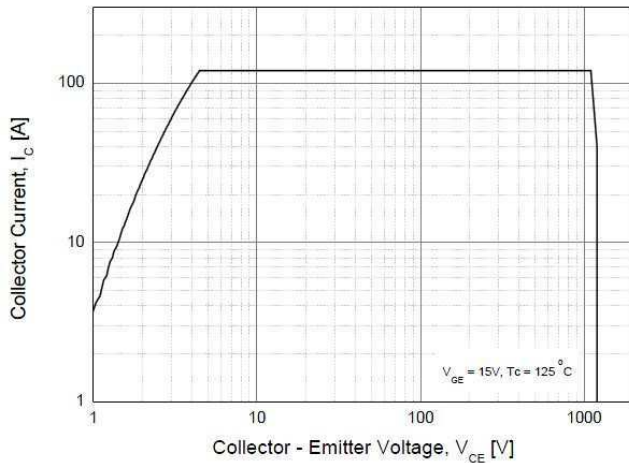
RBSOA
