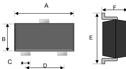
SOT-723
