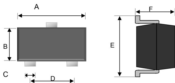
SOT-523
