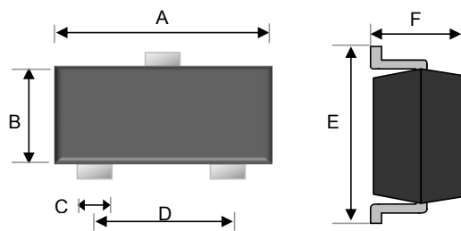
SOT-323
