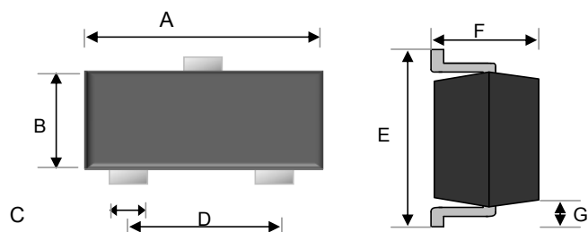
SOT-23
