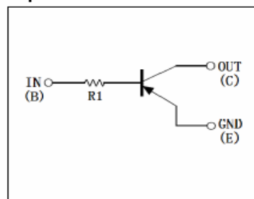
SOT-723/SOT-523 SOT-323/SOT-23
