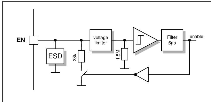
Figure 13 - EN input circuitry
