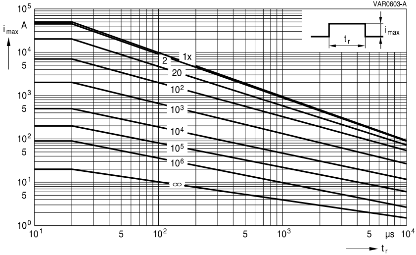
SIOV-LS41K130QP(K2) ... K150QP(K2)
