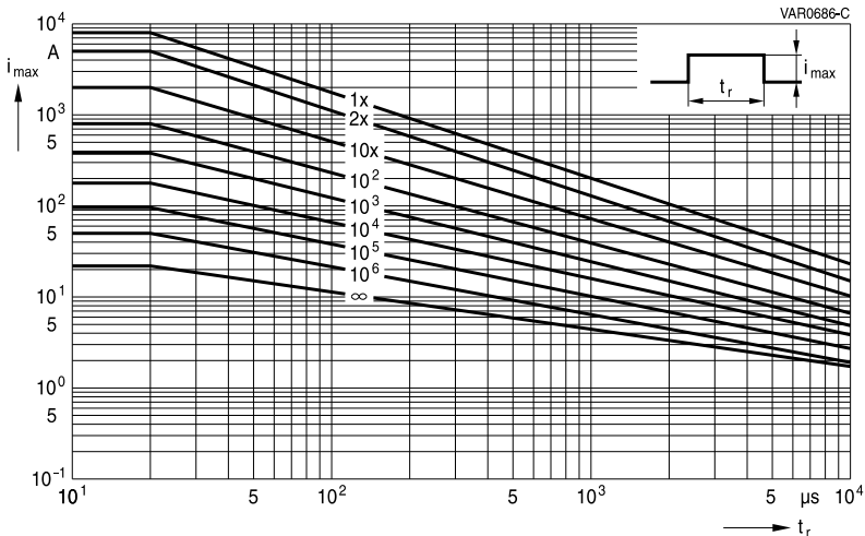
SIOV-Q14K350 ... K460
