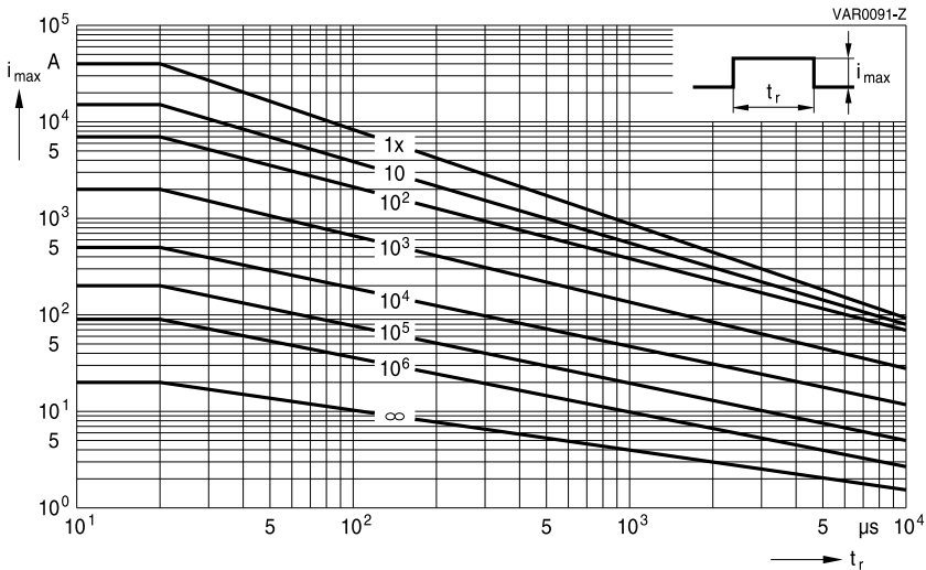
SIOV-B40K130 ... K150
