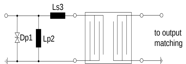
Fig. 2 Suppressor diode plus ESD matching
