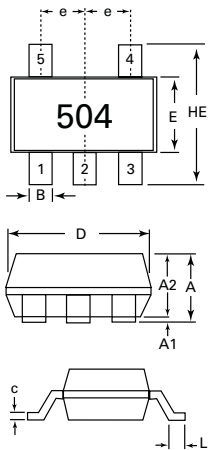
SP0504BAJTG - SC70-5
