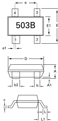
SP0503BAHTG - SOT143-4
