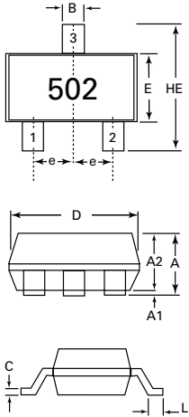
SP0502BAJTG - SC70-3
