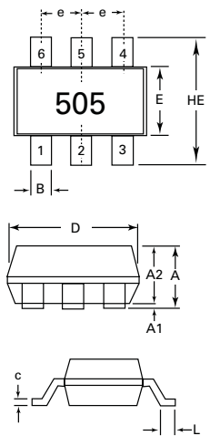
SP0505BAJTG - SC70-6
