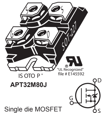
Single die MOSFET
