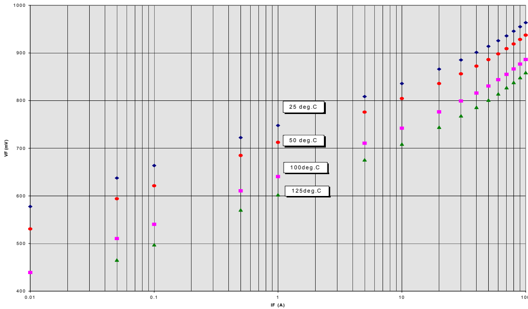
VF (IF) typical
