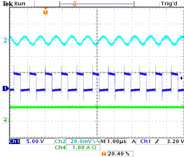
Fig. 10 - Output ripple
