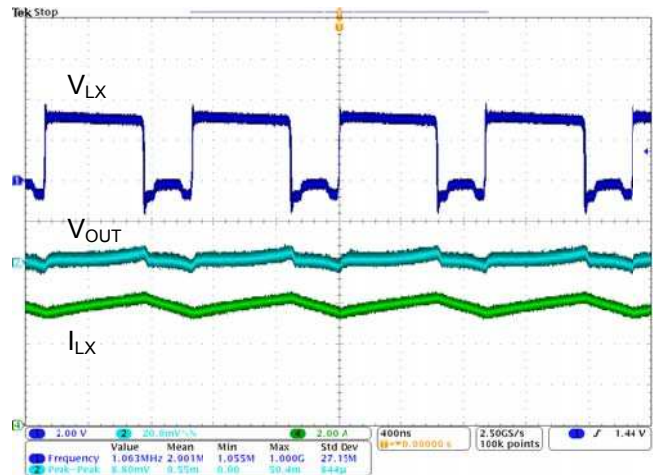
Fig.12 Output Ripple, Vin=3.3V, Vo=1.8V, Io=6A
