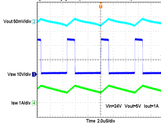
Output Ripple (24V→5V @1A)
