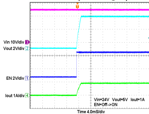
EN Off→ON Test (24V→5V @1A)
