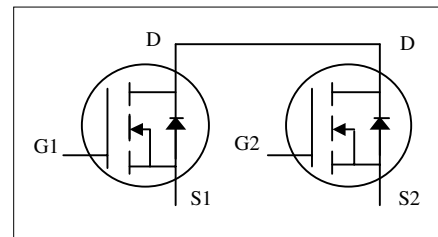
TSSOP-8
