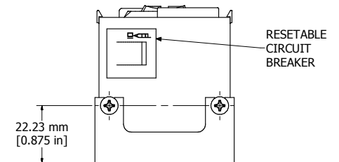
VIEW A-A
