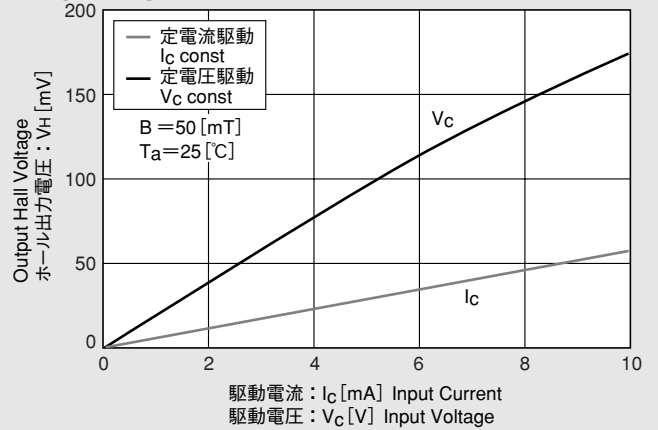
V_H-V_C, V_H-I_C
