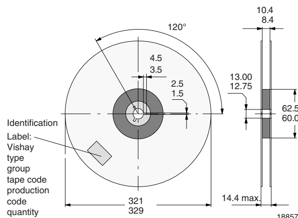
Fig. 25 - Reel Dimensions - GS18
