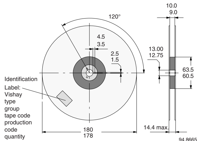
Fig. 24 - Reel Dimensions - GS08
