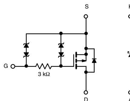
P-Channel MOSFET
