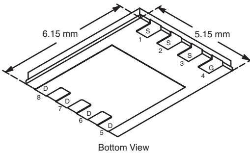
PowerPAK SO-8
