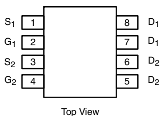
SO-8
