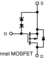
P-Channel MOSFET
