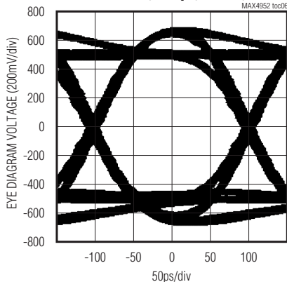
V_{IN} = 275mV_{p-p} , 6Gbps, PE = 1, EQ = 0
