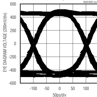
V_{IN} = 275mV_{p-p} , 6Gbps, PE = 0, EQ = 0
