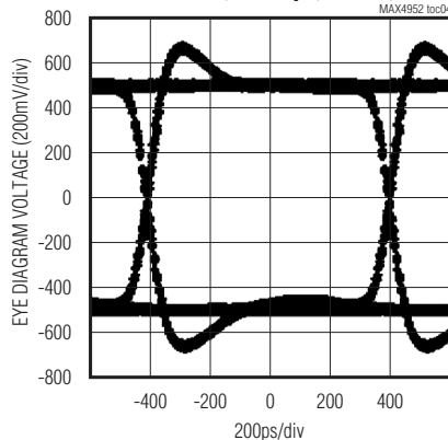
V_{IN} = 275mV_{p-p} , 1.5Gbps, PE = 1, EQ = 0
