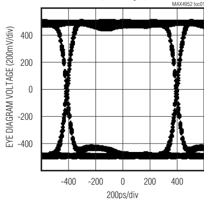
V_{IN} = 275mV_{p-p} , 1.5Gbps, PE = 0, EQ = 0
