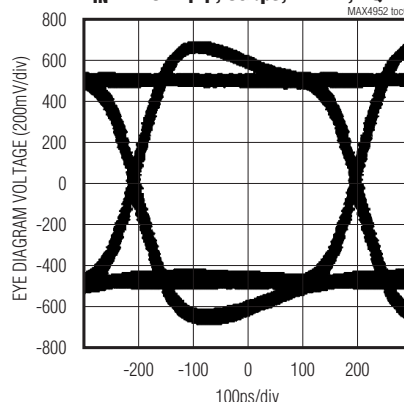
V_{IN} = 275mV_{p-p} , 3Gbps, PE = 1, EQ = 0
