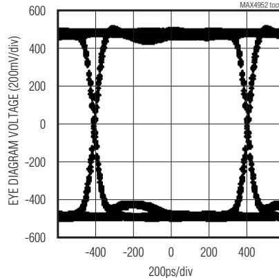
V_{IN} = 1600mV_{p-p} , 1.5Gbps, PE = 0, EQ = 0
