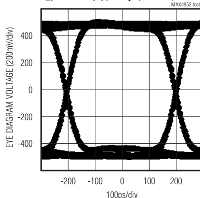
V_{IN} = 275mV_{p-p} , 3Gbps, PE = 0, EQ = 0
