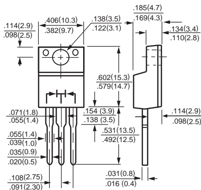
ITO-220
