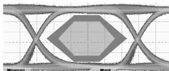
PRBS-23 Input @ 1.25Gbps, Optical
