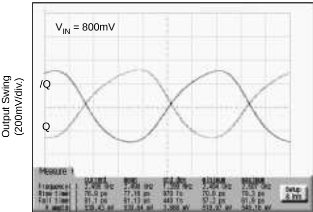
2.5GHz Output
