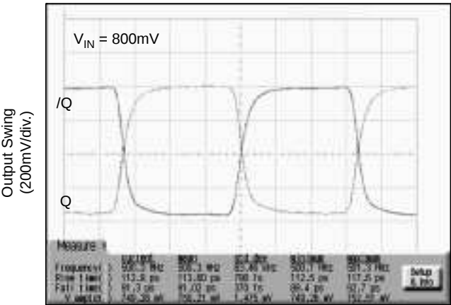
500MHz Output
