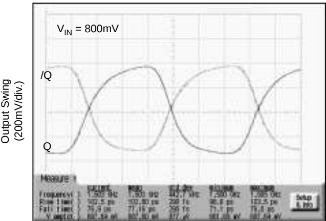
1.5GHz Output
