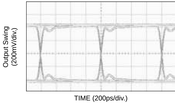
1.25Gbps Output (Q – I/Q)
