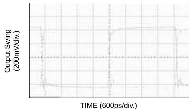
200MHz Output (Q – I/Q)
