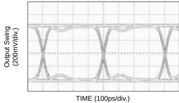
2.5Gbps Output (Q – I/Q)
