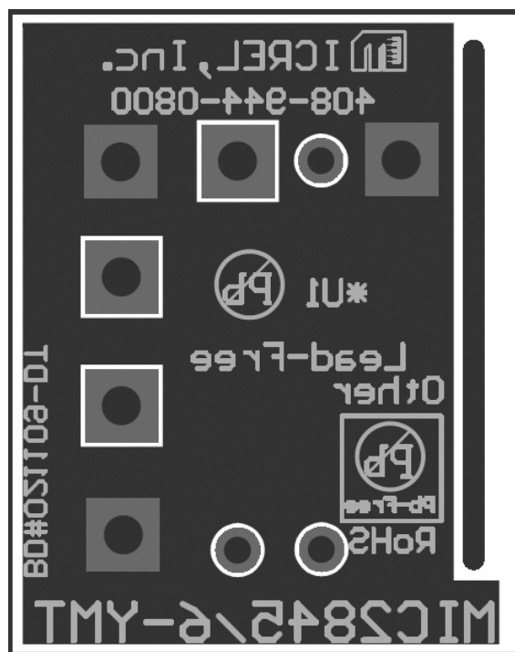
Bottom Layer
