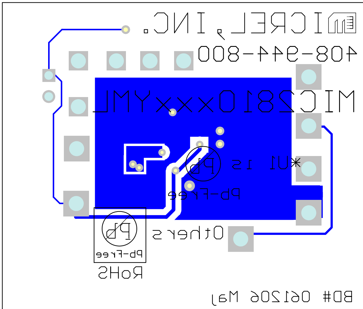
Bottom Layer
