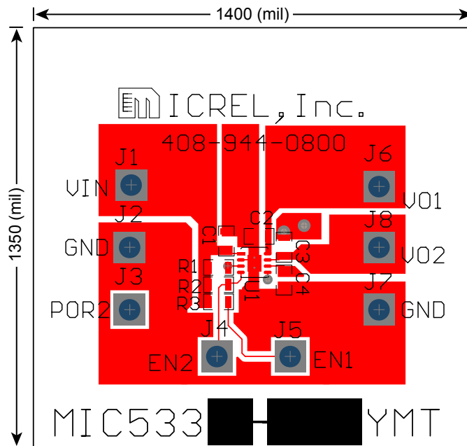
Top Layer
