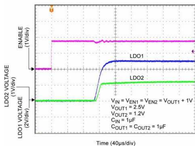
Enable Turn-On
