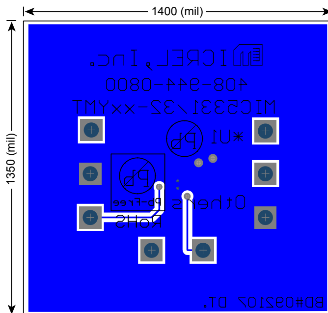
Bottom Layer
