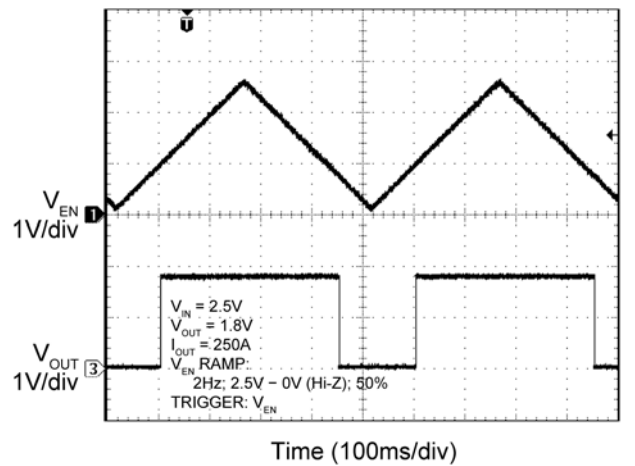
Enable Threshold
