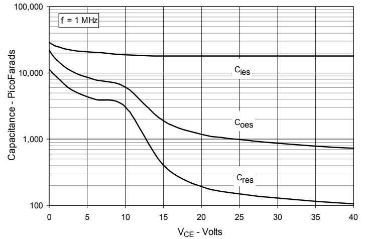
Fig. 8. Capacitance
