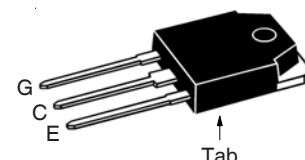
TO-3P (IXGQ)
