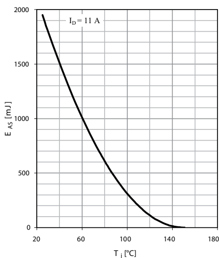
Fig. 10 Avalanche energy
