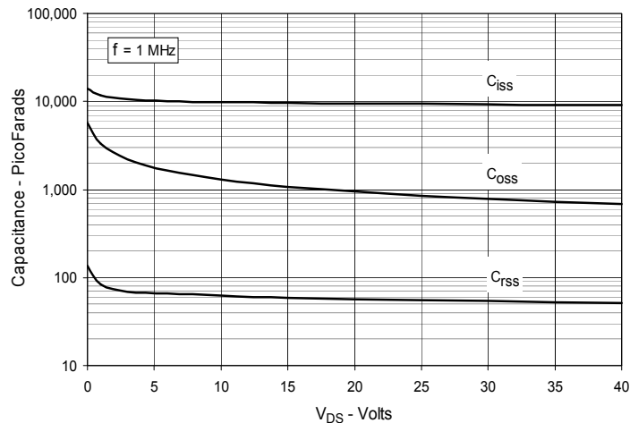
Fig. 11. Capacitance
