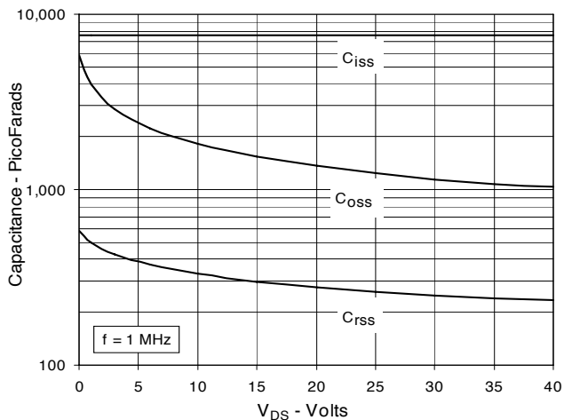
Fig. 11. Capacitance
