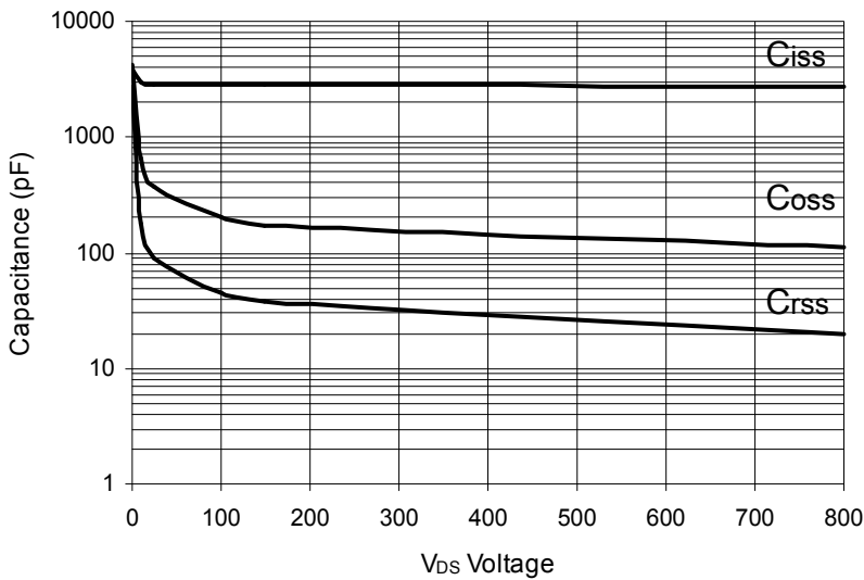
Fig. 5 V_{DS} vs. Capacitance
