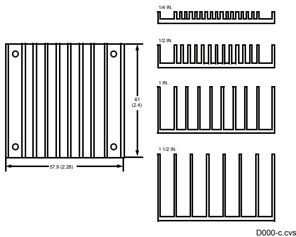
Figure 19. Longitudinal Heat Sink
