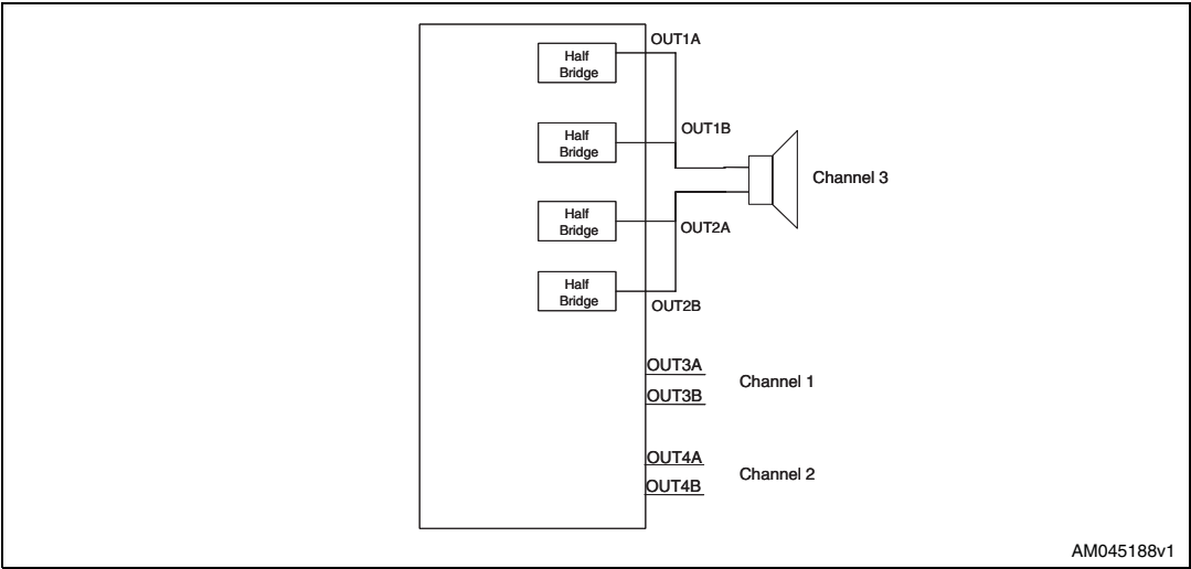
Figure 23. OCFG = 11
