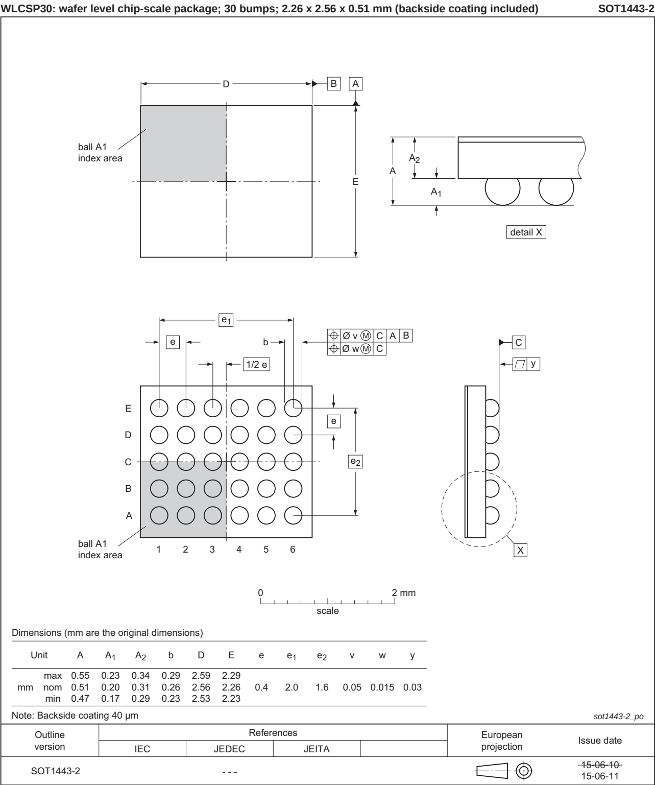
Fig 25. Package outline SOT1443-2 (WLCSP30)
