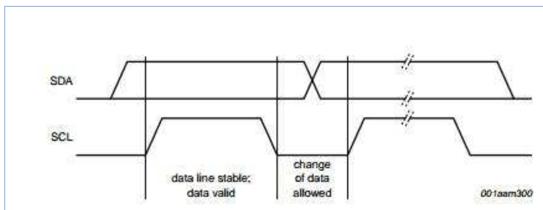
图 17. I2C 总线上的位传输
