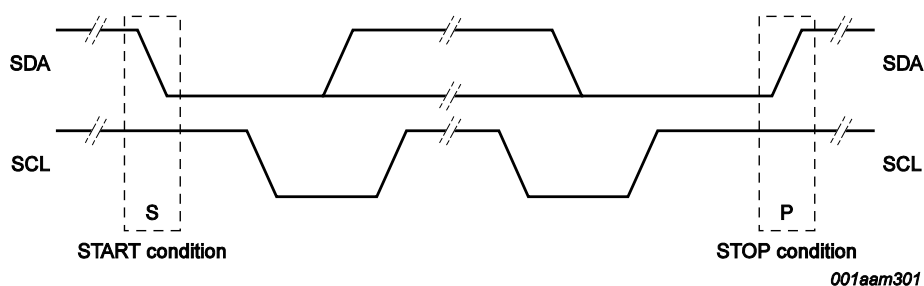
图 18. 起始和停止条件
