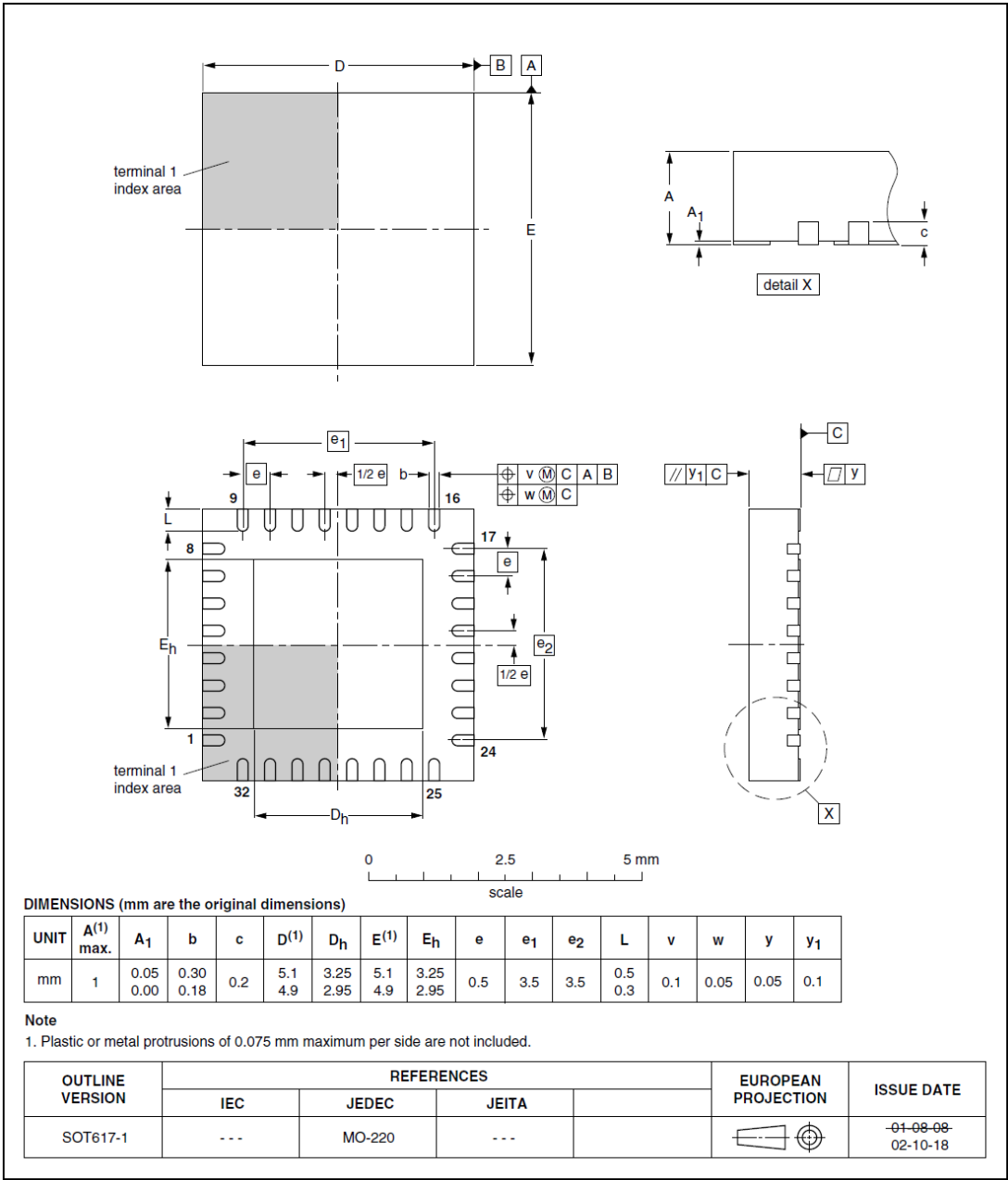
图 37. SOT617-1（HVQFN32）封装
