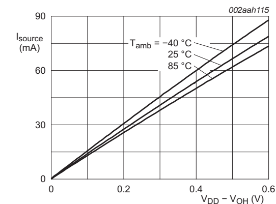
f. V_{\text{DD}} = 5.5\text{ V}
