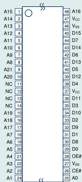
48TSOP(Type-I)
