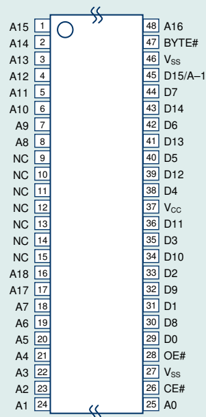
48TSOP(Type-I)
