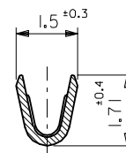
断面 A-A SECT. A-A
