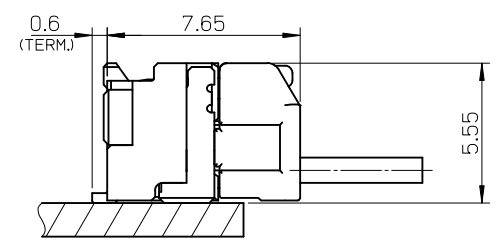
嵌合部 MATED CONNECTORS
