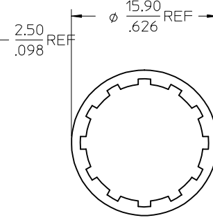
LOCKWASHER
