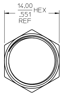
JAM NUT
