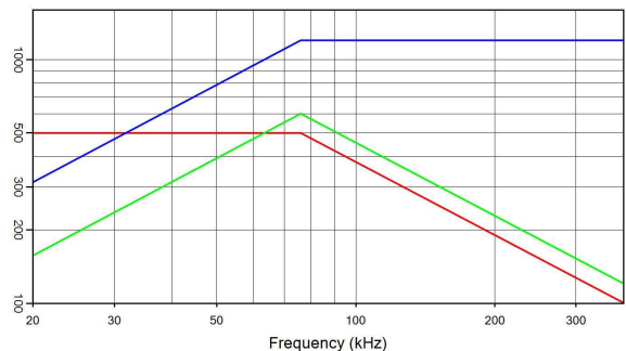
CSP305A/600 5 µF 500 V rms 1200 A rms 600 kVA r I(A) — Q(kVA r ) — V rms
