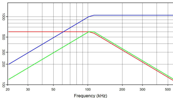
CSP305A/600 2.6 µF 600 V rms 1050 A rms 600 kVA r I(A) — Q(kVA r ) — V rms
