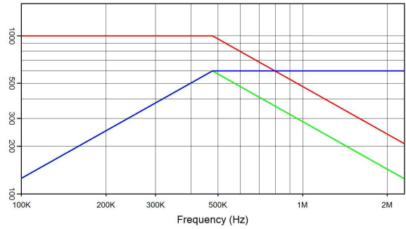
CSP305A/600 0.2 µF 1000 V rms 600 A rms 600 kVA r I(A) — Q(kVA r ) — V rms
