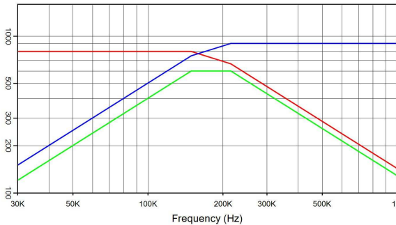
CSP305A/600 1 µF 800 V rms 900 A rms 600 kVA r I(A) — Q(kVA r ) — V rms
