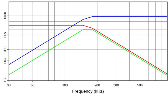
CSP305A/600 1.33 µF 700 V rms 950 A rms 600 kVA r I(A) — Q(kVA r ) — V rms
