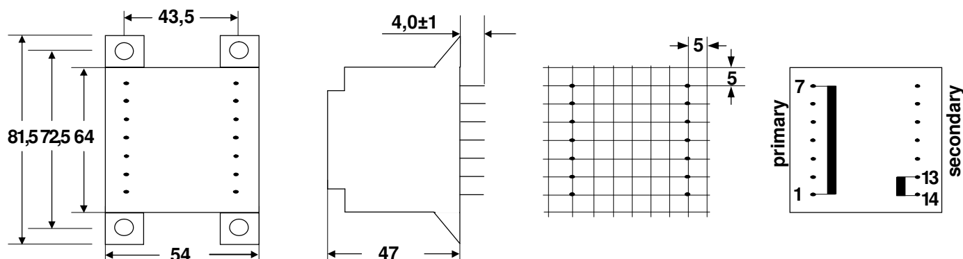
Abmessungen ±0,5mm / dimensions ±0,5mm / Ohne Maßstab / not scaled
