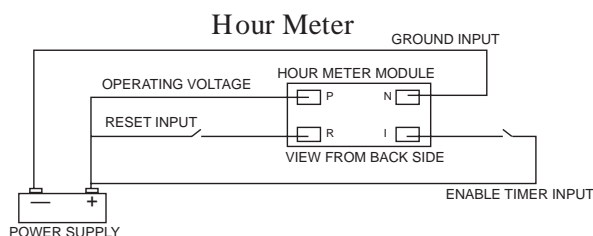
T1161AB Hour Meter
