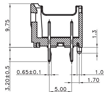
A-A Section
